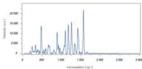
拉曼谱图
